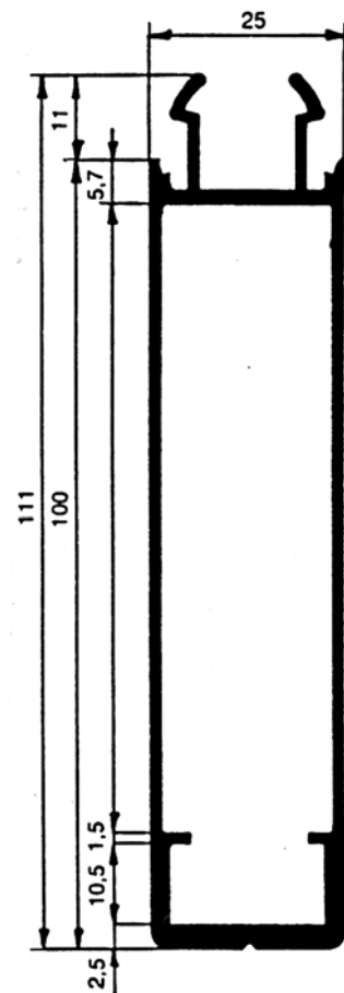
1122731 Undre kantprofil 1,370 kg/m
