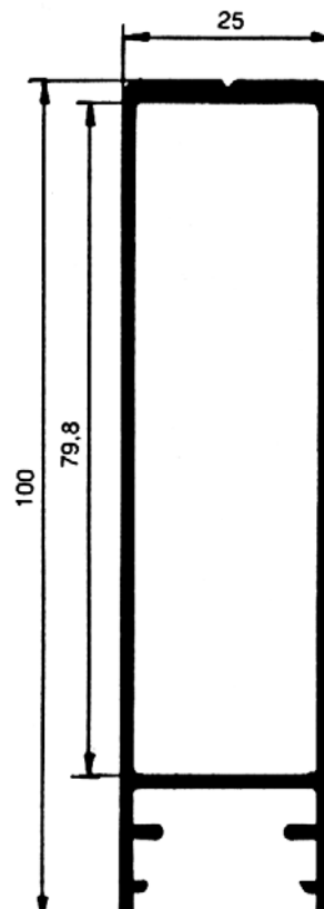
112278 Övre kantprofil 1,200 kg/m
