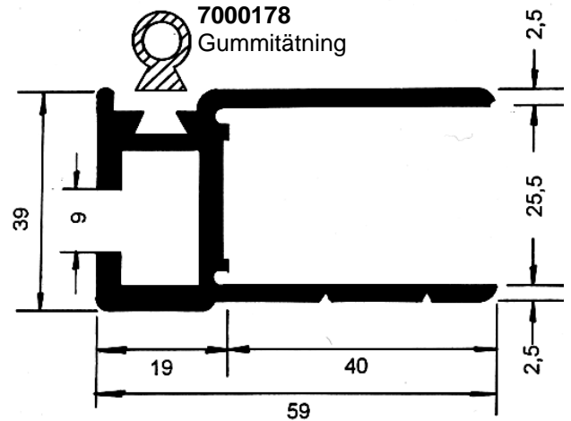
1140658 Kantskoning, anpassad till K1-K5 1,260 kg/m
