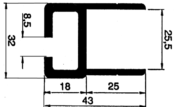
1400627 Kantskoning, anpassad till K1-K5 1,05 kg/m
