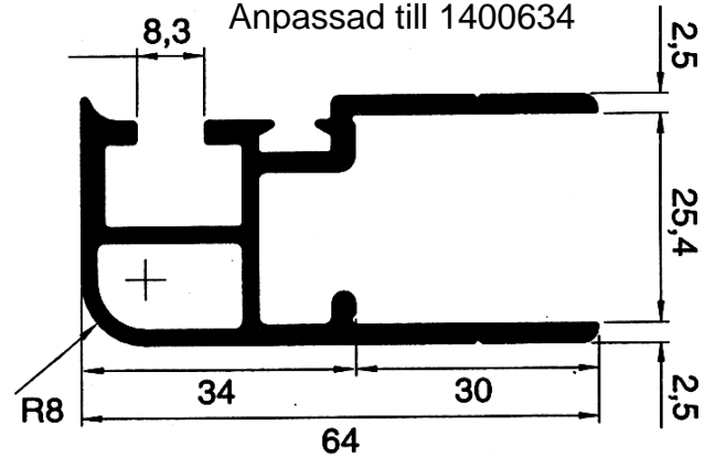
1400634 Kantskoning, anpassad till K20 1,20 kg/m
