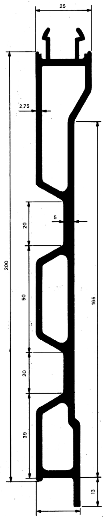
1123394 Undre kantprofil 3,656 kg/m
