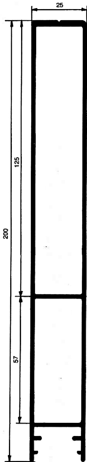
112277 Övre kantprofil 2,220 kg/m
