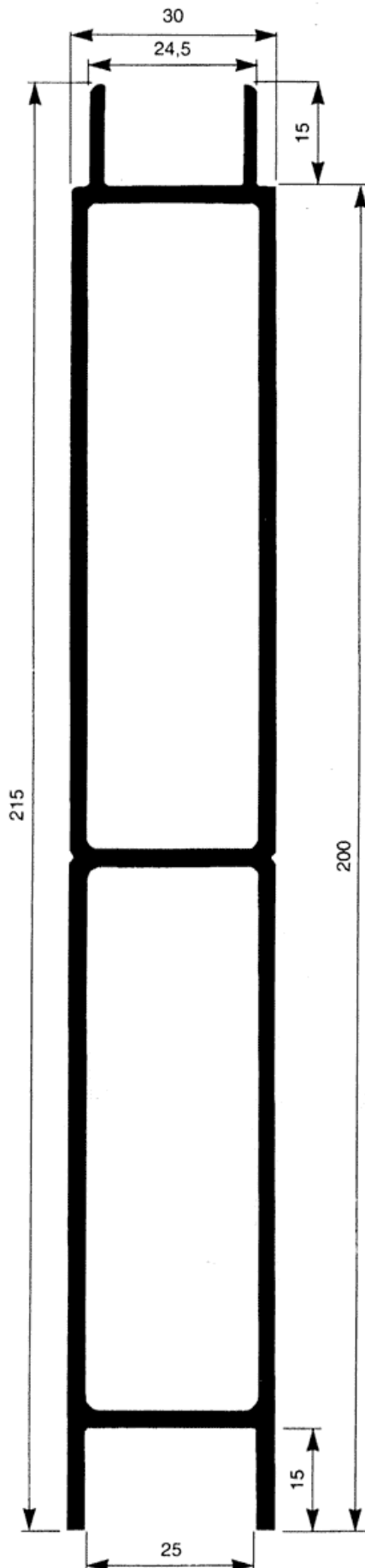
1120064 Mellanprofil 2,94 kg/m
