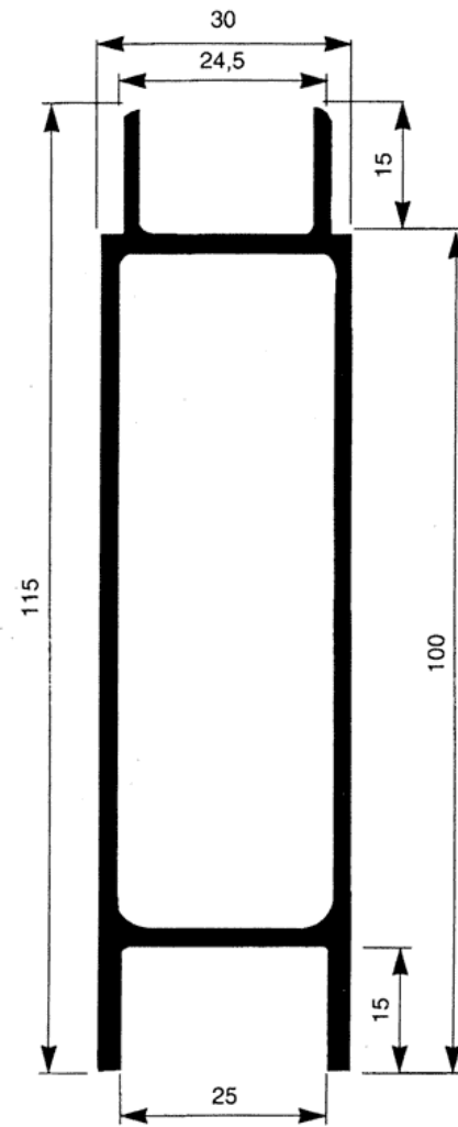
1120012 Mellanprofil 1,54 kg/m
