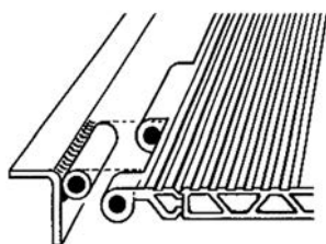
Alternativ 2 Påsvetsade stålrör
